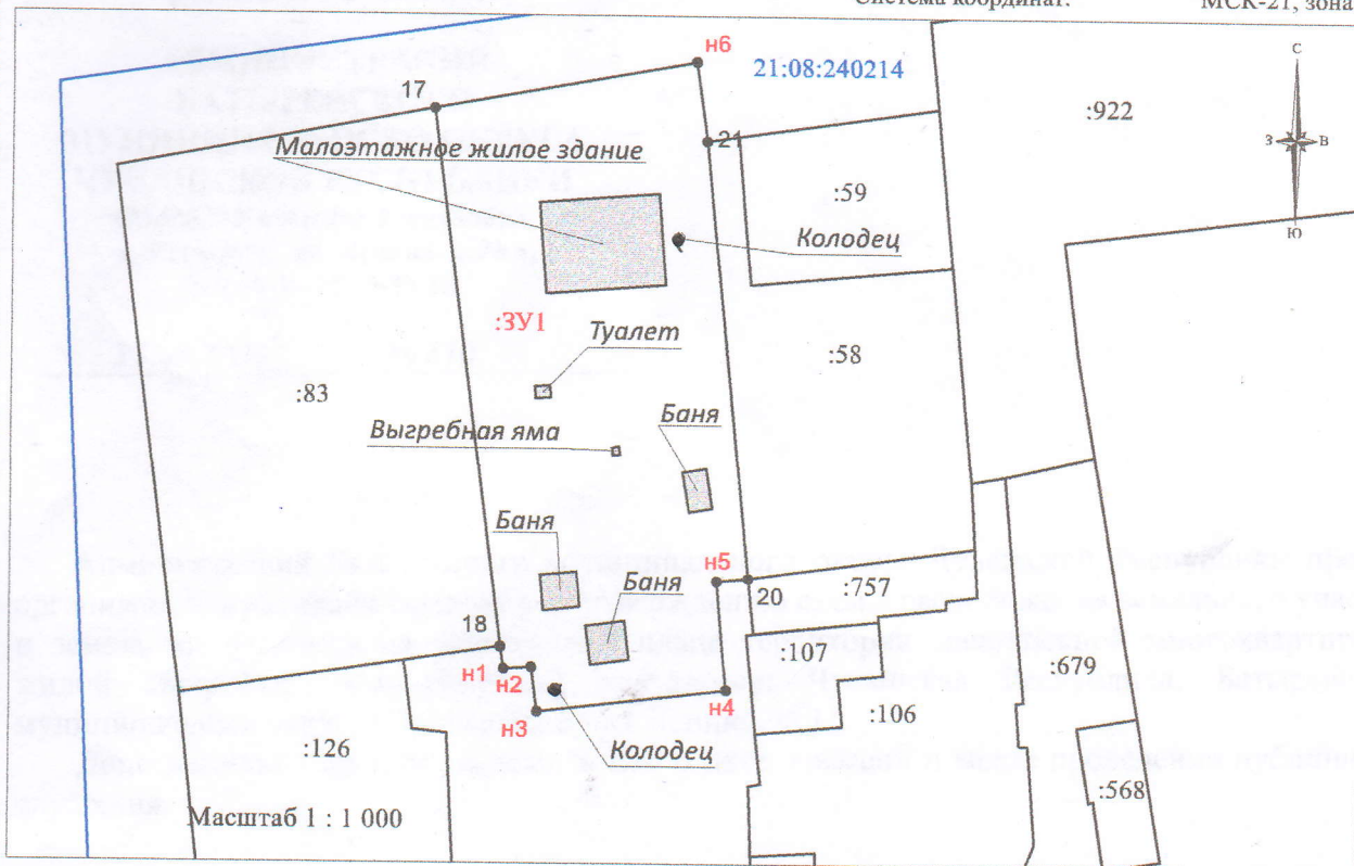
СИТУАЦИОННЫЙ ПЛАН
