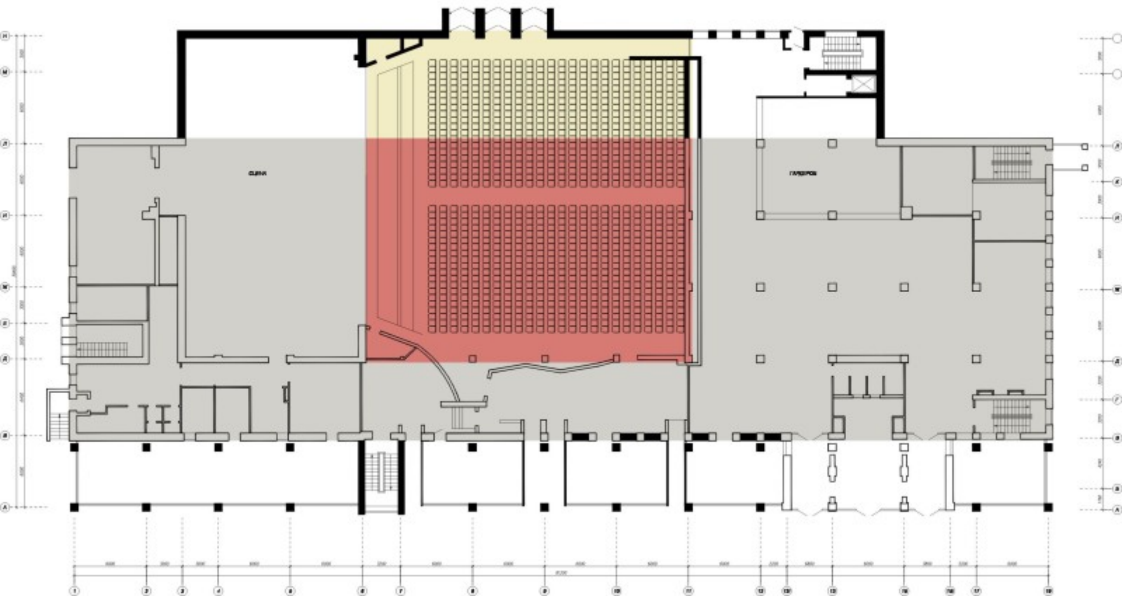
ПЛАН 1 ЭТАЖА
