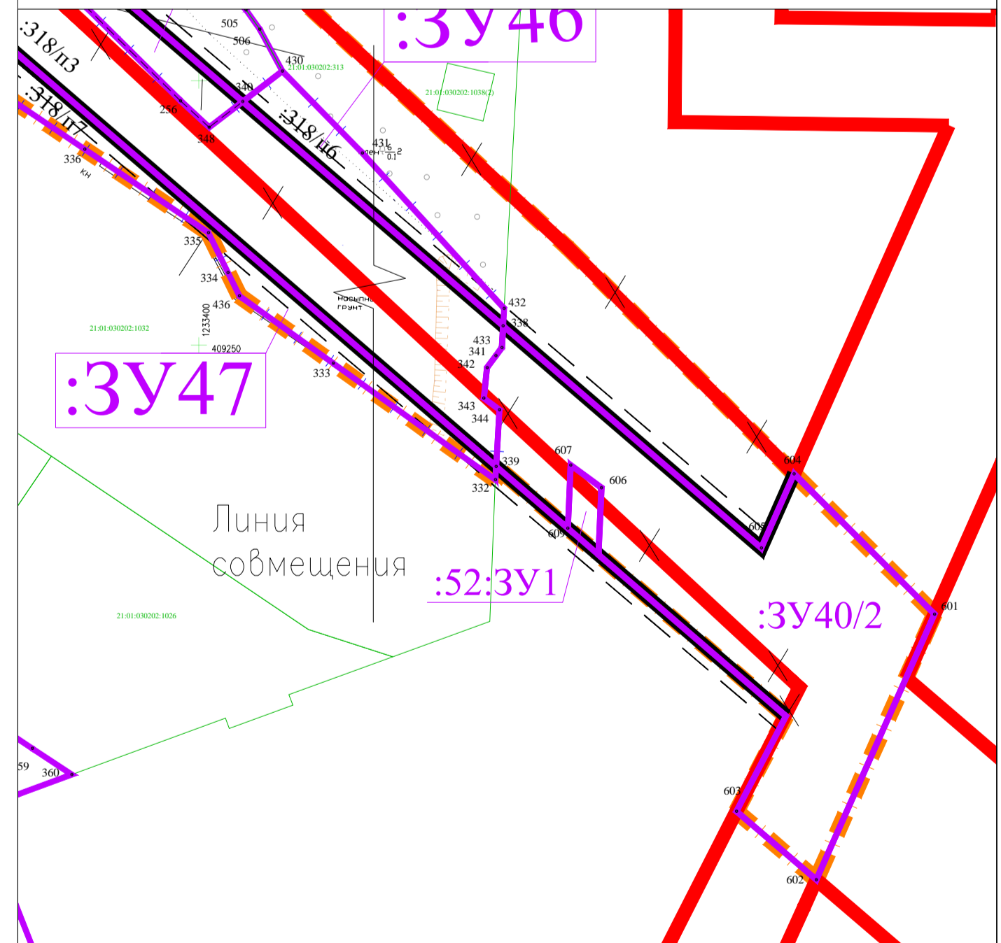
Фрагмент чертежа межевания территории
