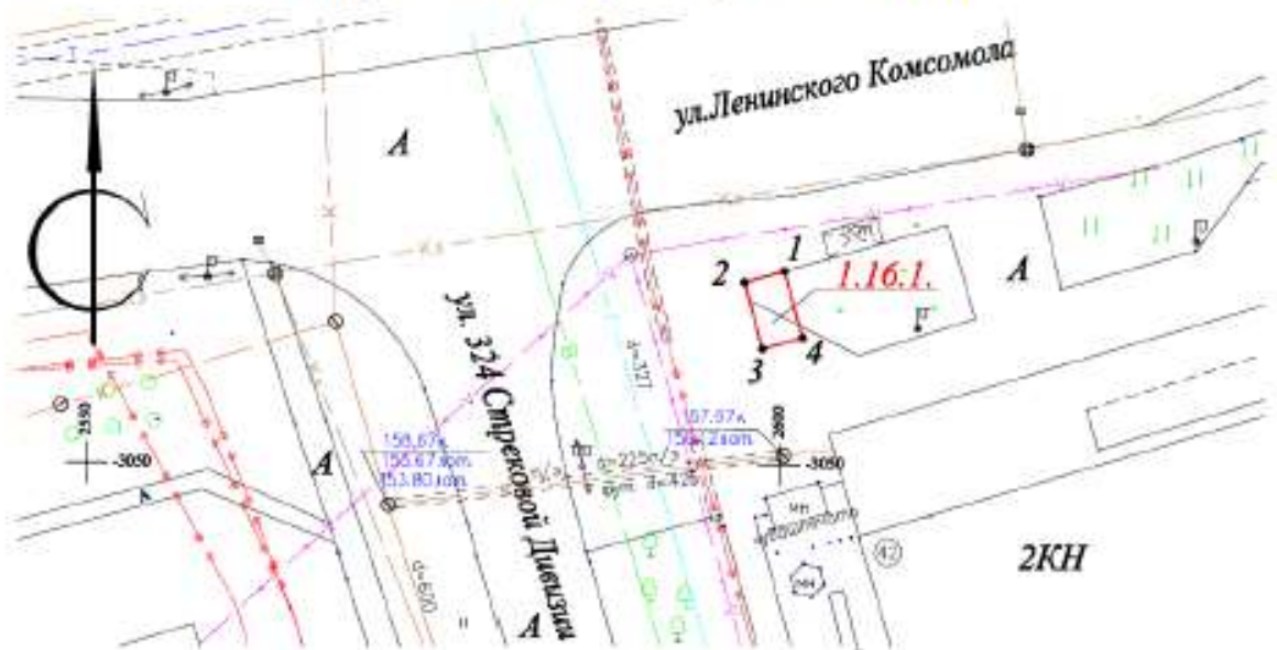
Схема размещения М 1:500
