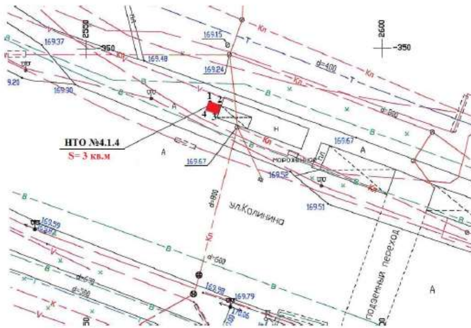
Схема размещения М 1:500
