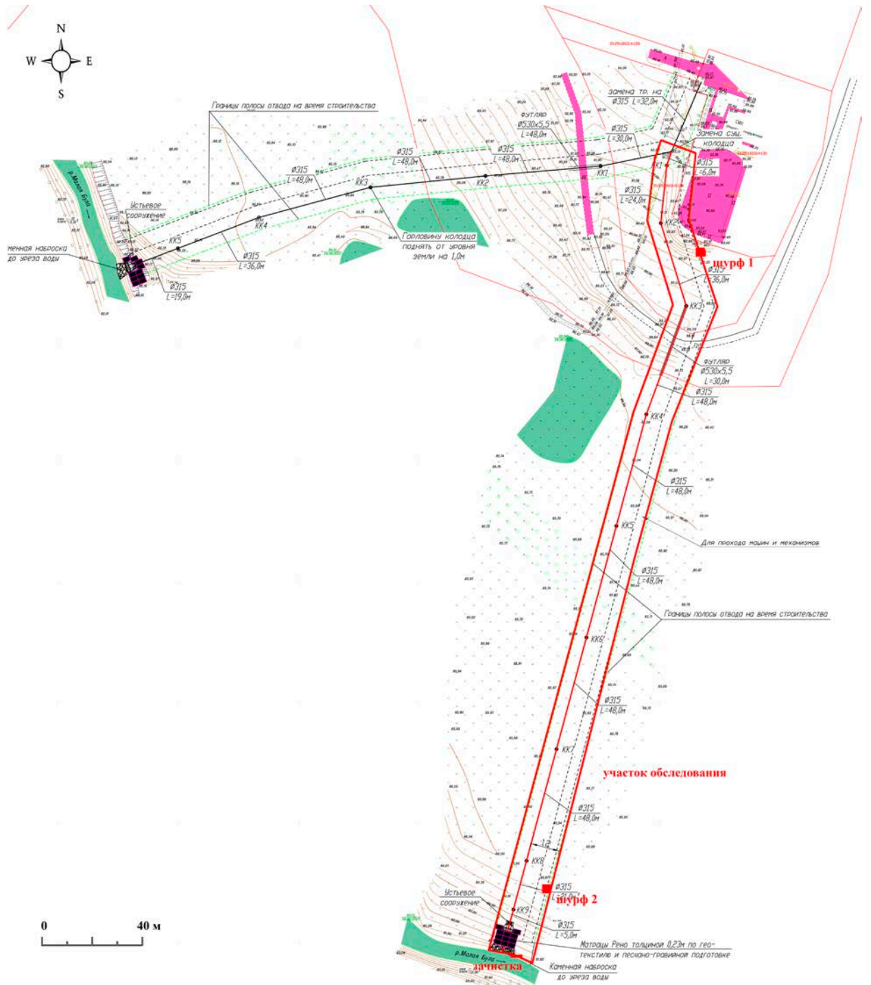
Илл. 3. Участок обследования в с. Яльчики Чувашской Республики. Район работ с указанием месторасположения шурфов и зачистки на инструментальном топографическом плане.
