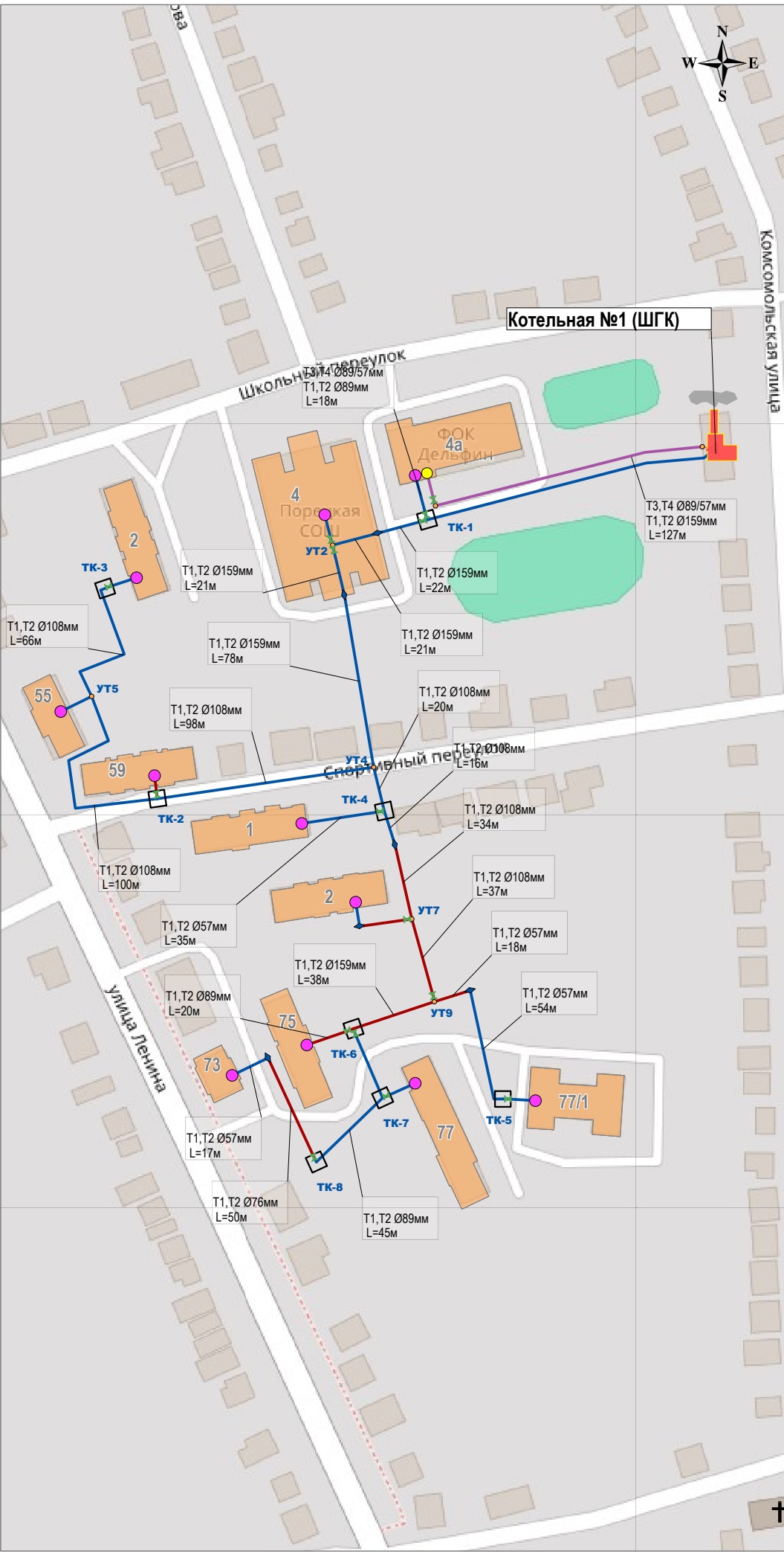
Приложение 5. Схема тепловых сетей от котельных Порецкого муниципального округа Чувашской Республики
