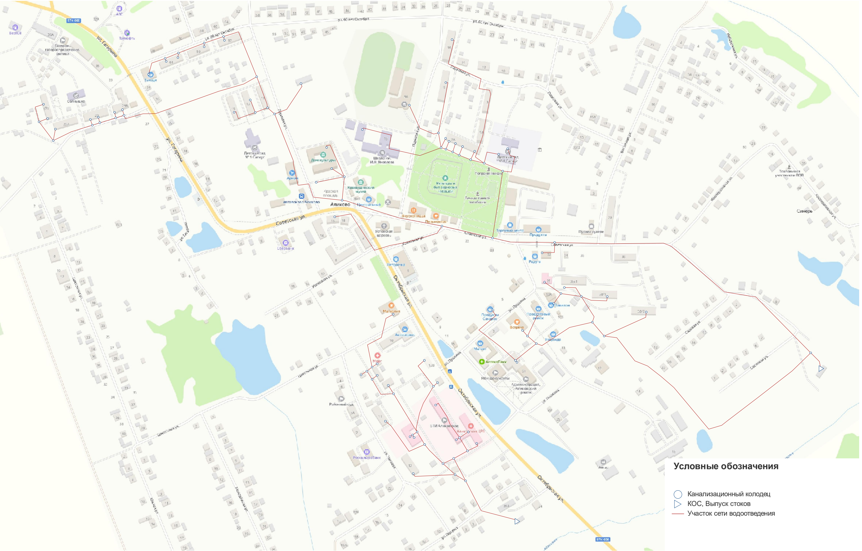
Приложение 46 - Схема сетей водоотведения с. Аликово
