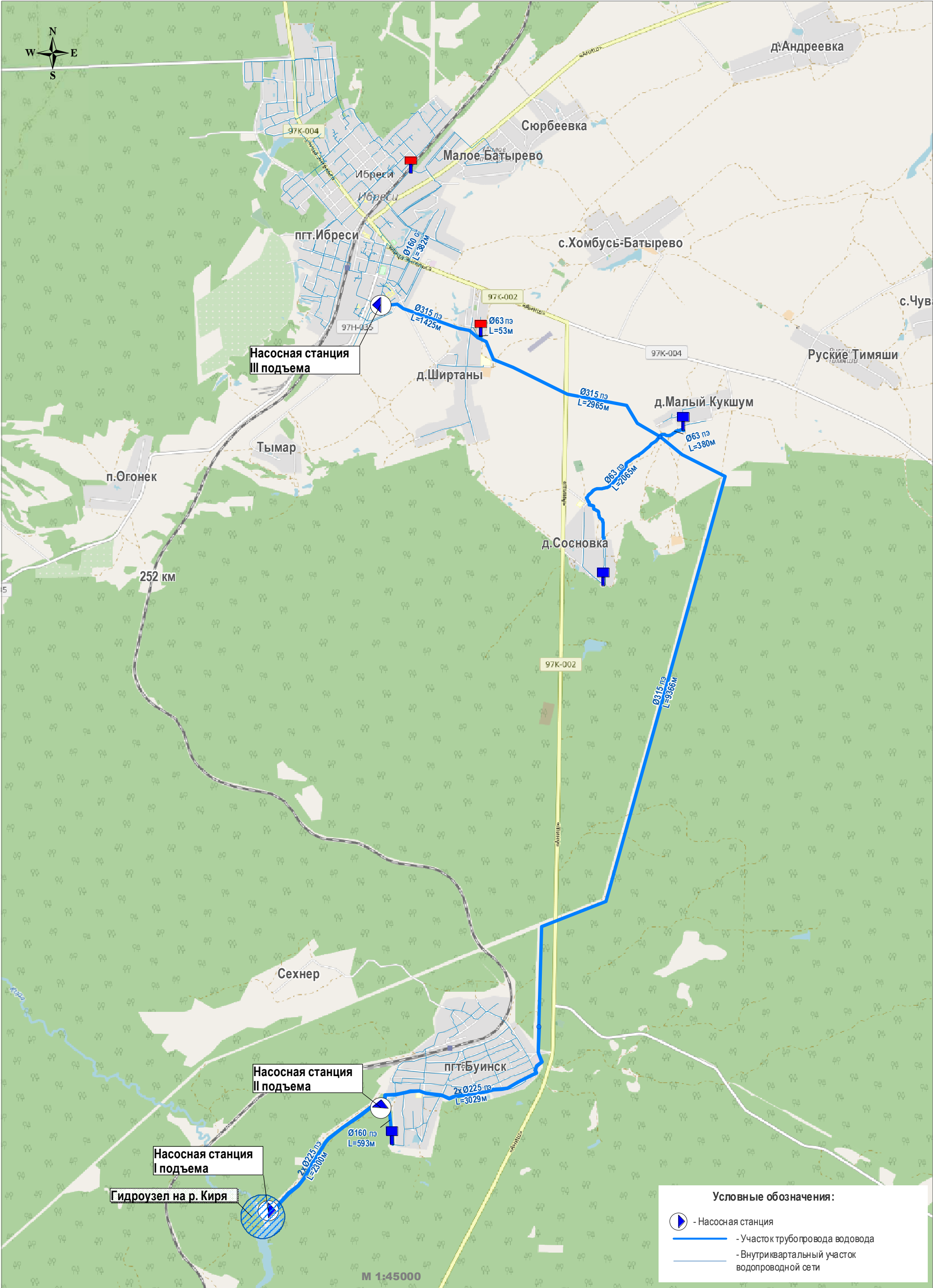
Приложение 1. Схема группового водовода от гидроузла на р.Киря до населенных пунктов Ибресинского муниципального округа Чувашской Республики
